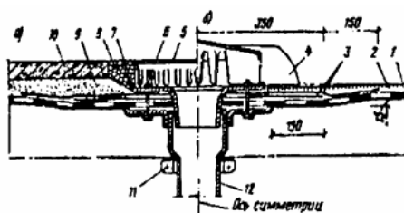
Ряс. 4. Примеры решения кровель в местах установки водосточных воронок
