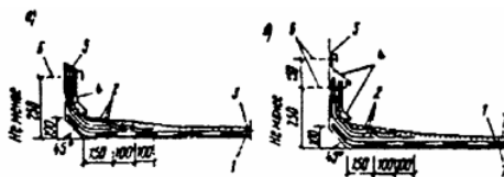
Рис. 1. Примеры примыканий кровель
