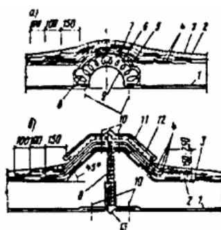
Рис. 7. Примеры решений деформационных швов
