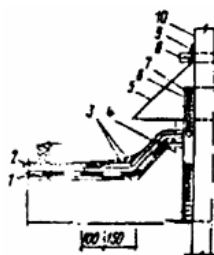
Рис. 3. Пример решения пропуска труб
