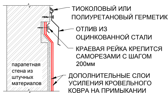
Рис. 24 Заведение края кровельного ковра под выдру в парапетной стене.
