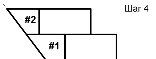
Рис. 9. Раскрой и расположение теплоизоляционных плит в не прямых углах кровли.
