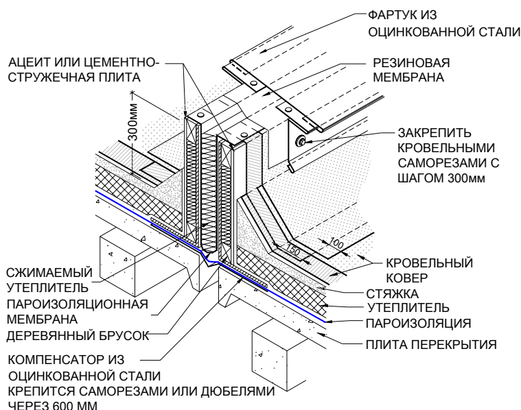
Рис. 5. Деформационный шов.
