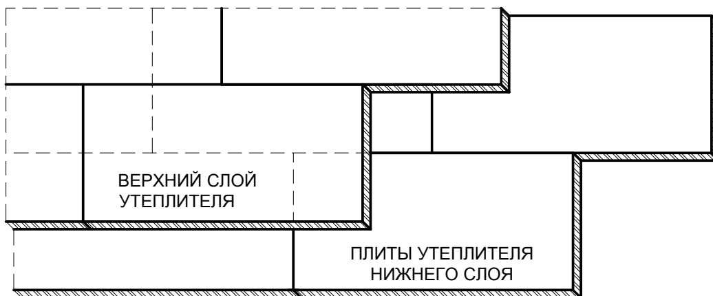
Рис. 7. Смещение плит верхнего и нижнего слоев при укладке.
