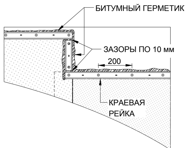
Рис. 22. Оформление края ковра краевой рейкой.
